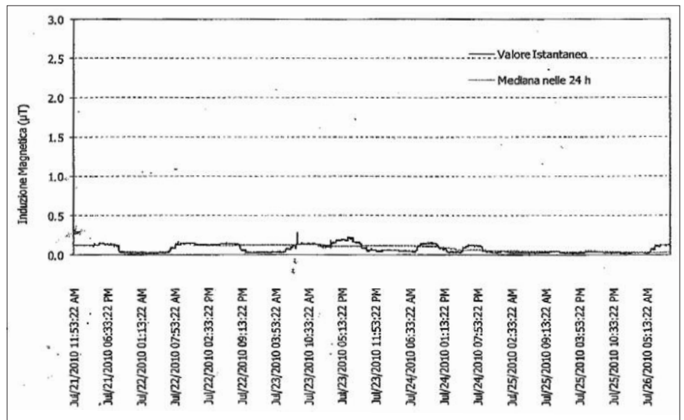
Grafico 1: Andamento del valore di campo induzione magnetica registrato con Emdx Lite a intervalli di 60 secondi e andamento della corrispondente mediana calcolata nelle 24 ore.
